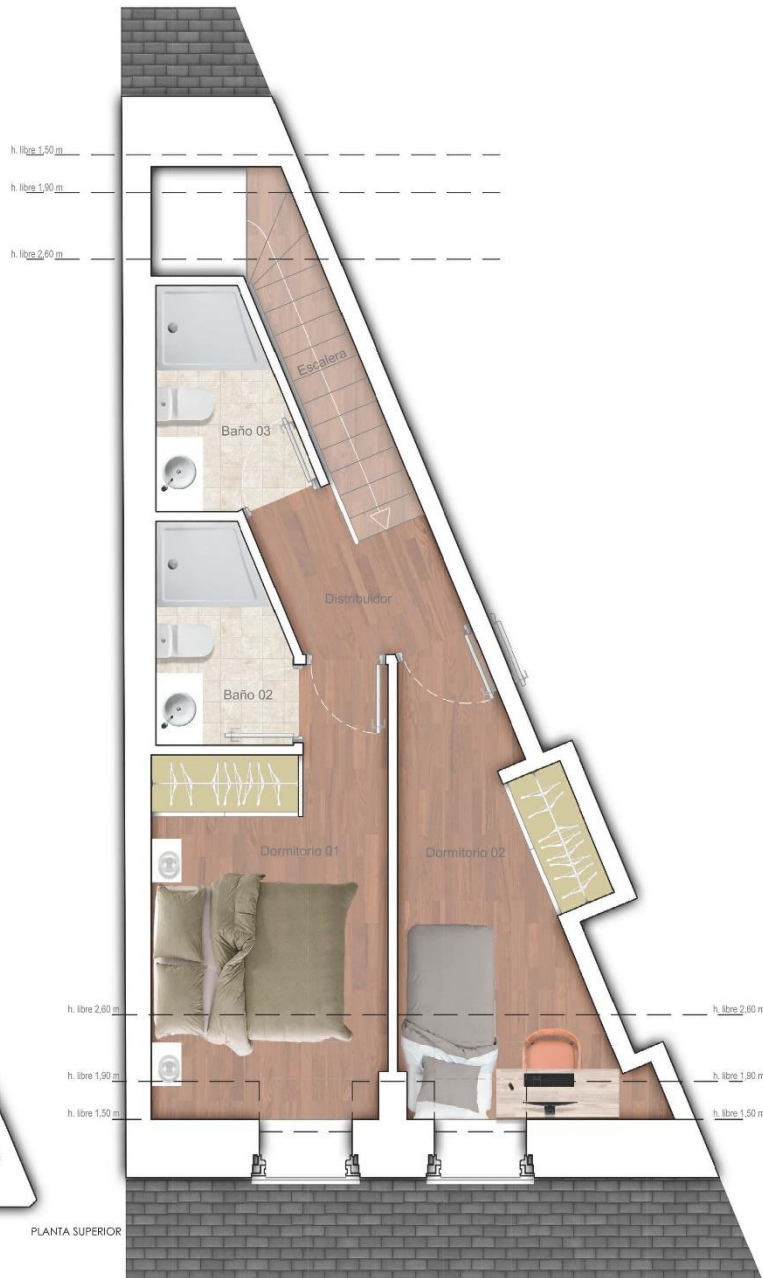
PLANTA INFERIOR
